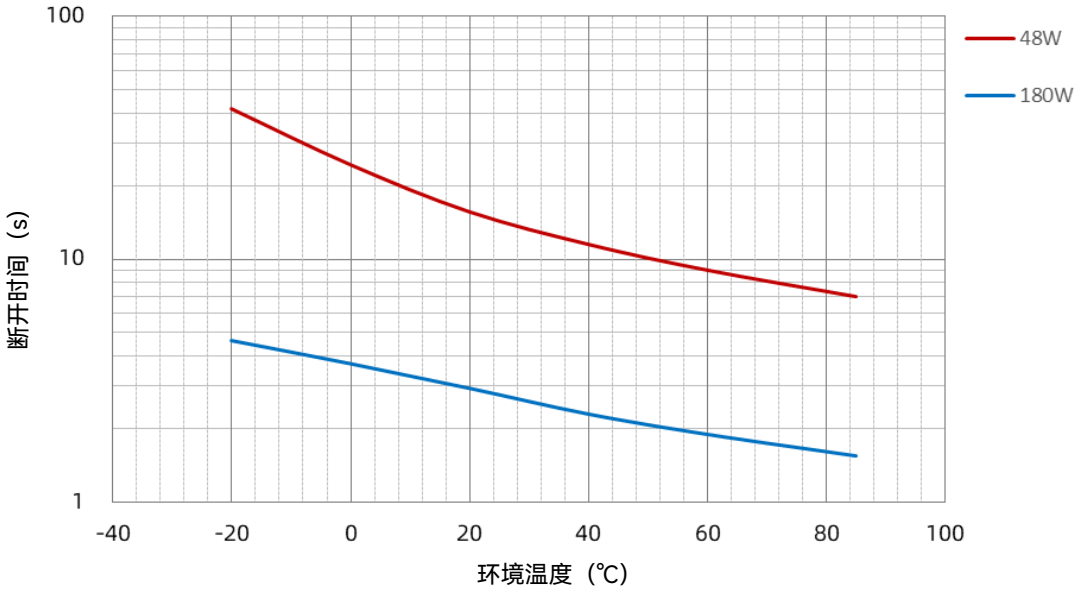
SKT-L 150 A 功率-温度曲线
