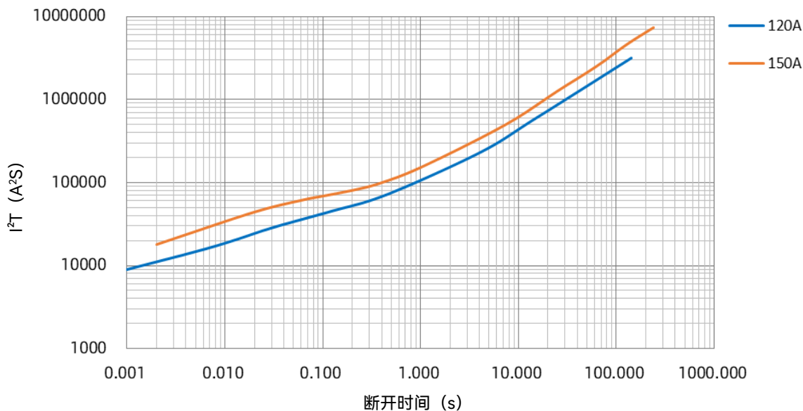
SKT-L I^2t -t 曲线
