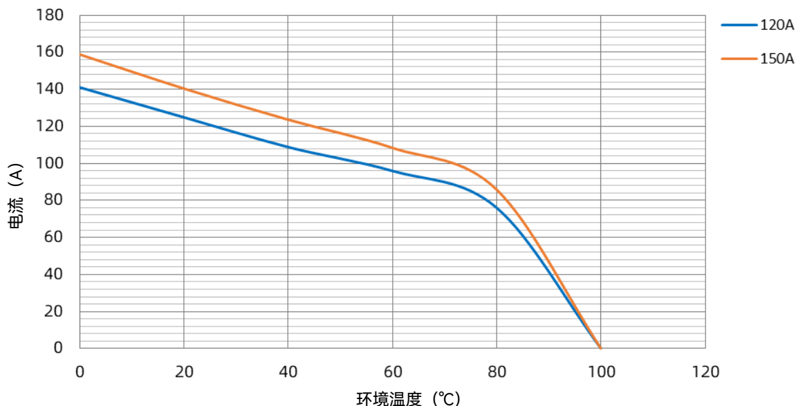
SKT-L 载流能力曲线
