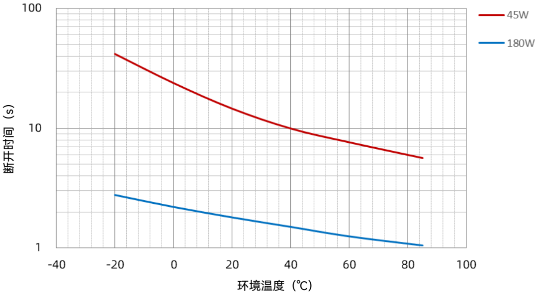
SKT-L 120 A 功率-温度曲线
