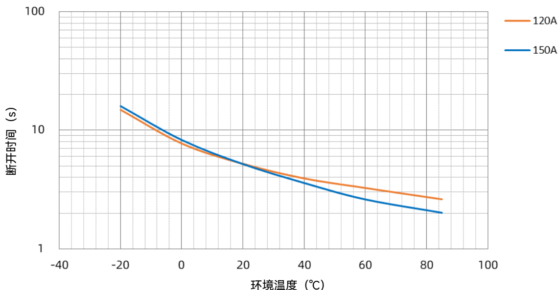
SKT-L 温度-时间曲线
